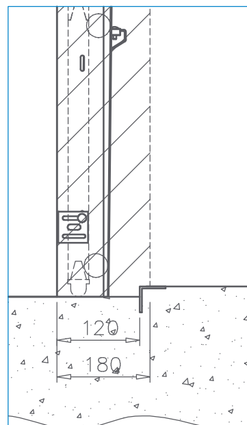
DETAIL A: WATERKERING
